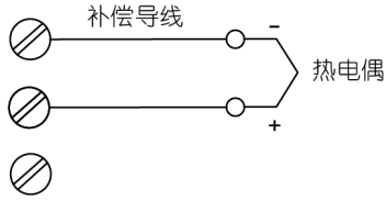
(1) 内部自动补偿模式 (补偿导线应直接接到接线端子上)
